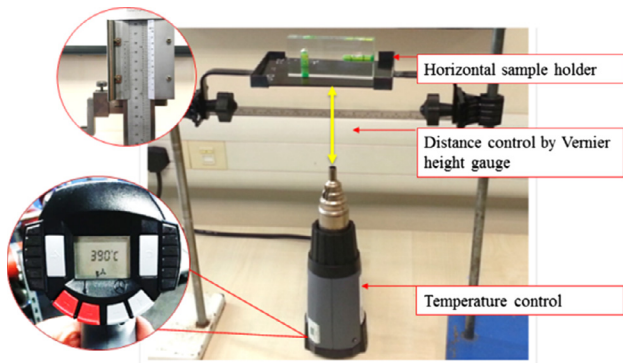
Fig. 1. Heat exposure test rig.
