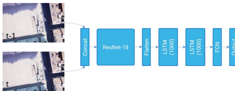
Figure 8: CNN-LSTM VO
