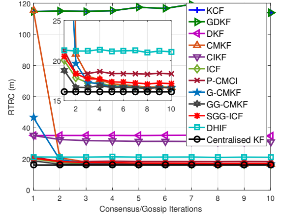
(b) RTRC
